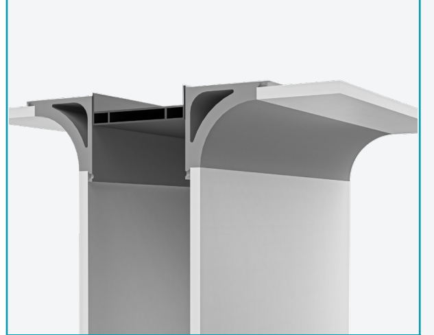
Duvar ve Tavan Bağlantısı Alüminyum Birleşim Profili
